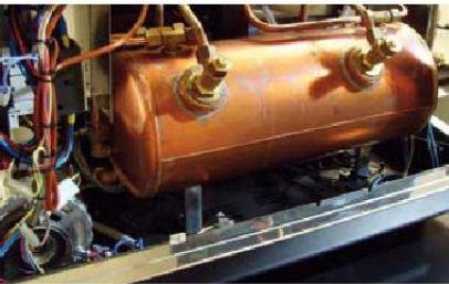
Interior de una máquina de espresso donde se visualiza, al centro la caldera y a la izquierda la bomba.
