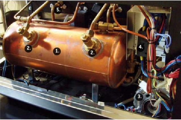
1. Caldera 2. Intercambiadores de calor 3. Bomba y motor 4. Tarjeta controladora 5. Sistema hidráulico.
